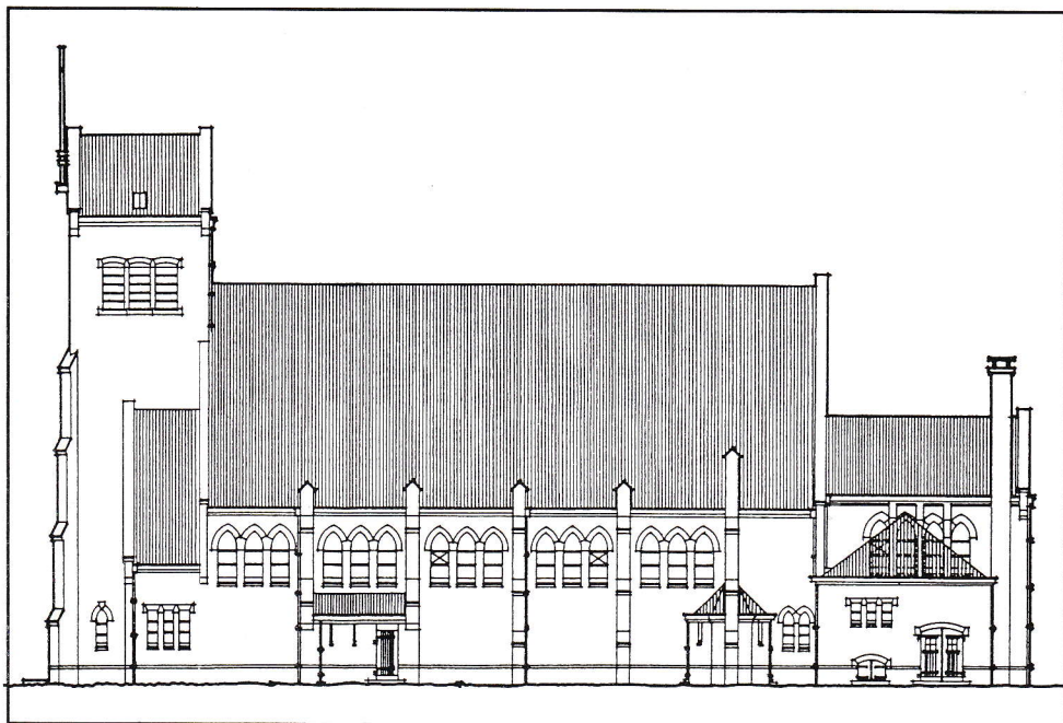
De zuidwestelijke gevel van de rooms-katholieke kerk aan de Nassaulaan op de ontwerptekening uit 1933. De architect van deze kerk, Jan van Dongen, bouwde in een stijl die verwant is aan het traditionalisme. Gebruikmakend van traditionele materialen als baksteen, natuursteen en hout wordt veel aandacht besteed aan het monumentale aspect. Bij dit gebouw wordt dat ondermeer duidelijk bij de geaccentueerde ingangspartij met een belangrijke rol voor de diagonaal geplaatste steunberen (Rijksarchief in Drenthe, archief Rooms-Katholieke parochie Maria ten Hemelopneming)
