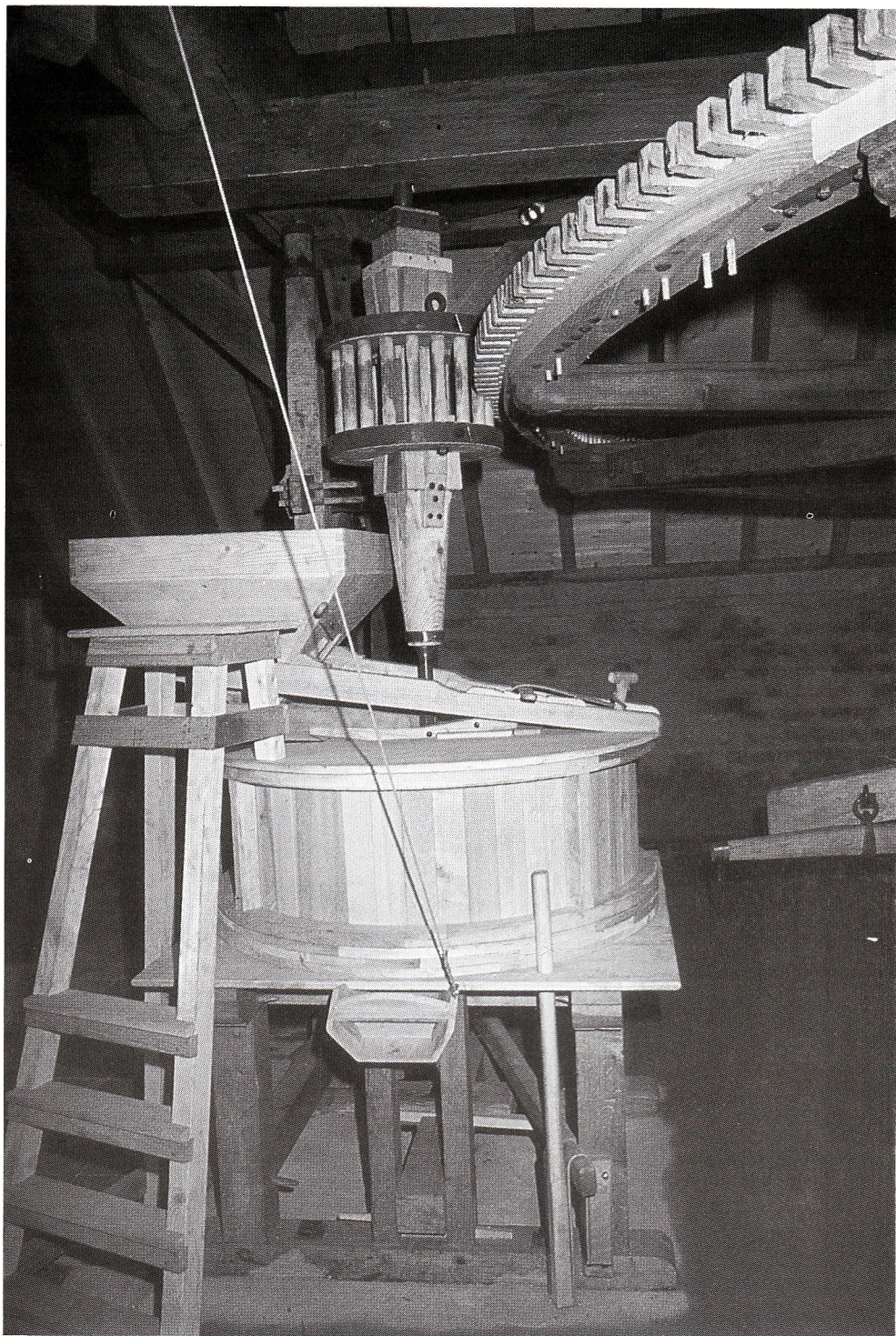
Het centrale deel van de koren-rosmolen te Zeddam. In het ronde houten omhulsel bevinden zich de maalstenen. Het koren werd er linksboven ingegooid, gemalen door de maalstenen en kwam als mer' weer tevoorschijn uit de schuif die onder het maalgedeelte te zien is (foto Ir. A.J. IJzerman, 1974).
